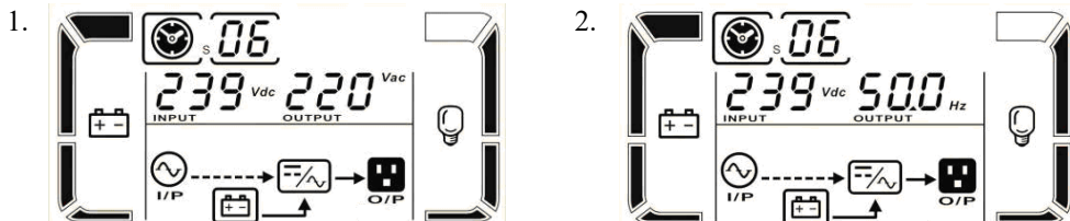
Рисунок 18 – Показания LCD-дисплея ИБП в режиме тестирования батарей
