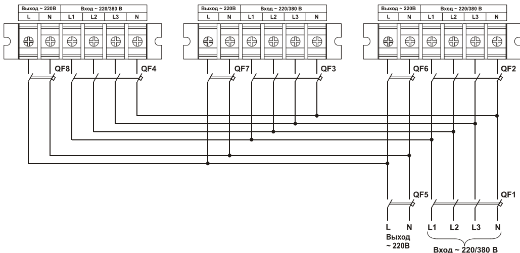
Рисунок 26 – Соединение входов и выходов трех ИБП в параллельной системе
