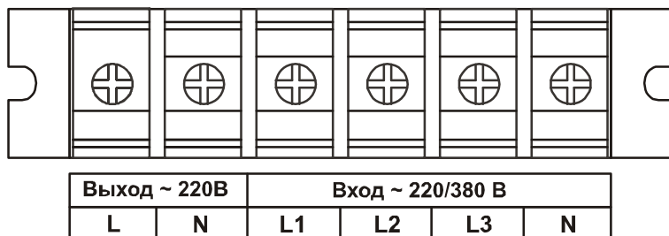
Рисунок 5 – Внешний вид клеммного блока ИБП ATS 10000 3/1 T-X (R)
