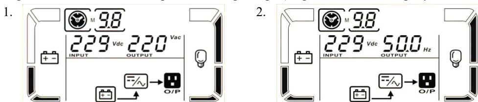
Рисунок 16 – Показания LCD-дисплея ИБП в автономном режиме
