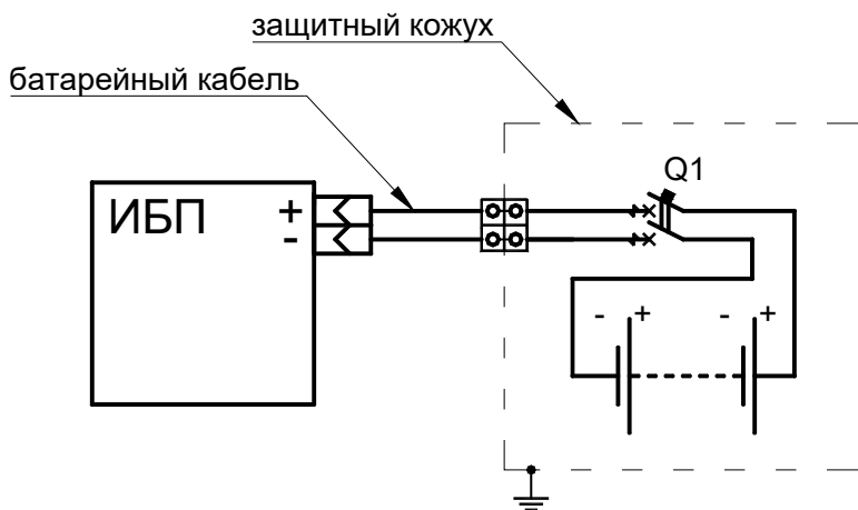
Рисунок 7 – Схема электрическая подключения аккумуляторов к ИБП
