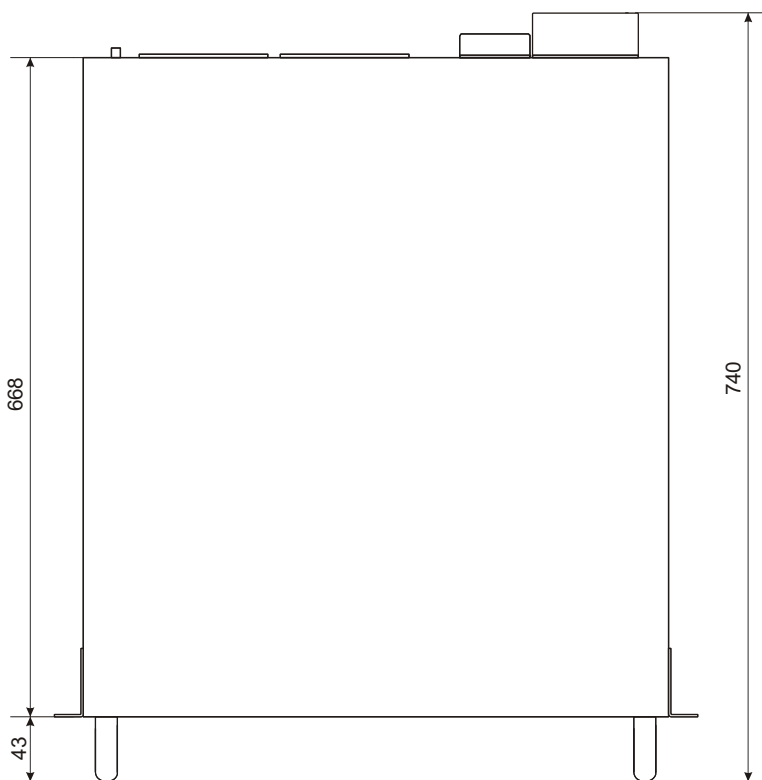
Рисунок А.2 – Габаритные и установочные размеры ИБП «ATS 15000 3/1 T-X(R)» и «ATS 20000 3/1 T-X(R)»
