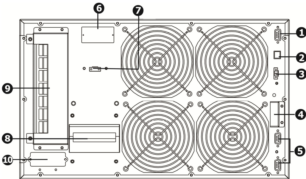
Рисунок 4 - Задняя панель ИБП ATS 15000 3/1 T-X (R), ATS 20000 3/1 T-X (R)
