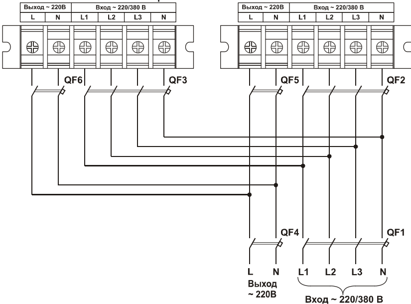
Рисунок 25 – Соединение входов и выходов двух ИБП в параллельной системе
