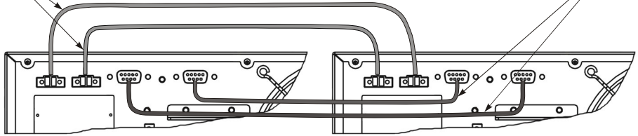
Рисунок 23 – Подключение информационных кабелей к двум ИБП в параллельной системе
