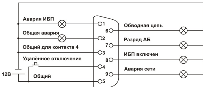
Рисунок 10 – Электрическая схема организации контроля и управления ИБП с электропитанием от источника постоянного тока напряжением +12 В
