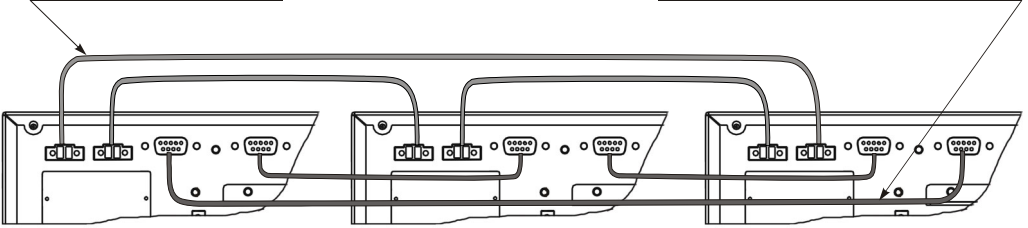
Рисунок 24 – Подключение информационных кабелей к трем ИБП в параллельной системе
