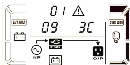
Рисунок 20 – Показания LCD-дисплея ИБП с кодами предупреждающих сообщений
