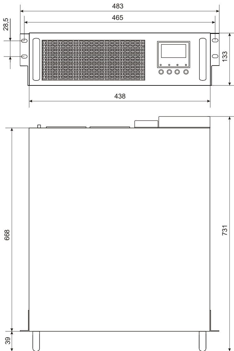
Рисунок А.1 – Габаритные и установочные размеры ИБП «ATS 10000 3/1 T-X(R)»
