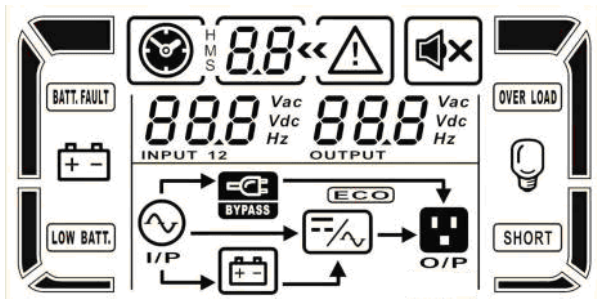
Рисунок 12 – Показания LCD-дисплея ИБП при включении
