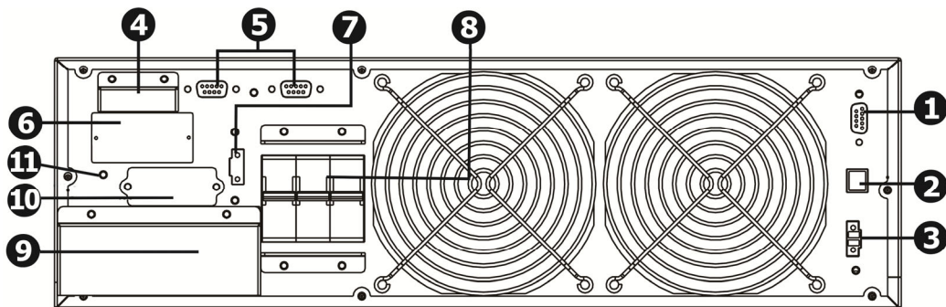
Рисунок 3 - Задняя панель ИБП ATS 10000 3/1 T-X (R)
