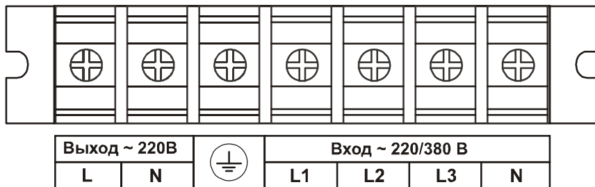
Рисунок 6 – Внешний вид клеммного блока ИБП ATS 15000 3/1 T-X (R), ATS 20000 3/1 T-X (R)
