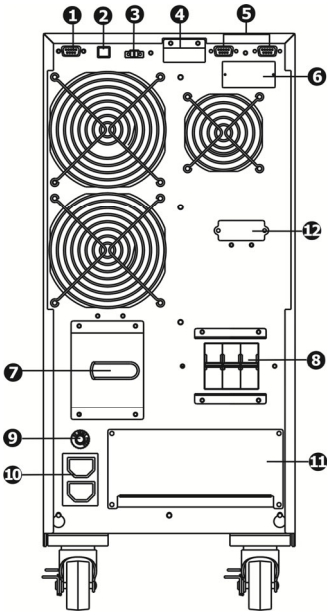
Рисунок 3 - Задняя панель ИБП ATS 10000 3/1 T-BX, ATS 10000 3/1 T-X
