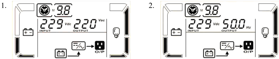
Рисунок 21 – Показания LCD-дисплея ИБП в автономном режиме
