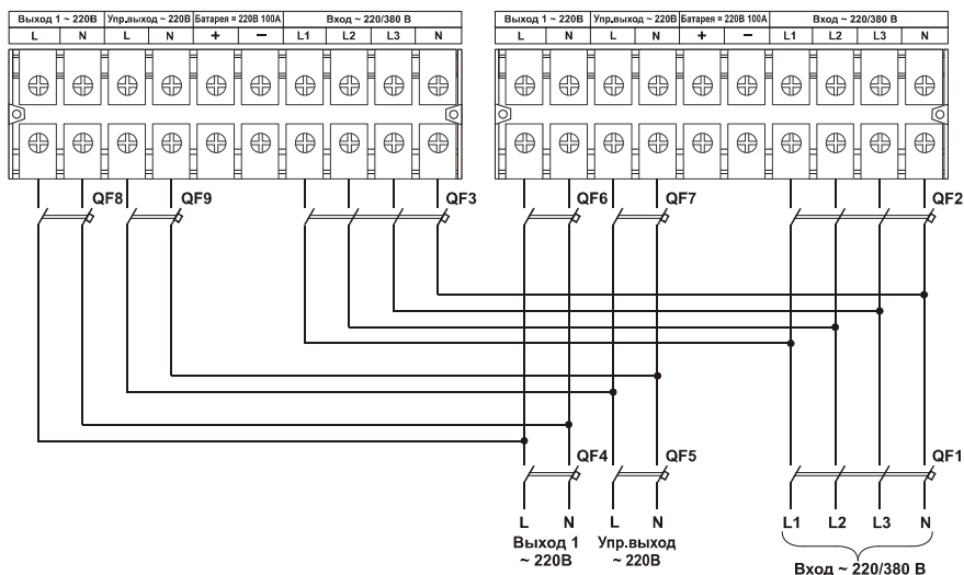
Рисунок 30 – Соединение входов и выходов двух ИБП в параллельной системе
