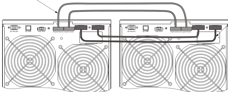
Рисунок 28 – Подключение информационных кабелей к двум ИБП в параллельной системе
