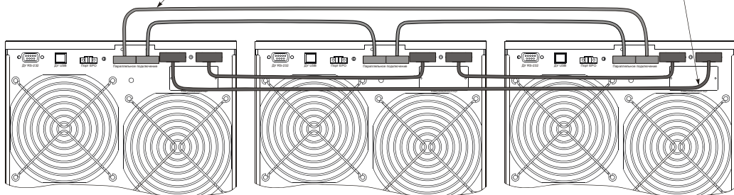
Рисунок 29 – Подключение информационных кабелей к трем ИБП в параллельной системе
