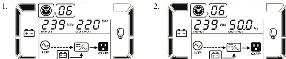
Рисунок 23 – Показания LCD-дисплея ИБП в режиме тестирования батарей
