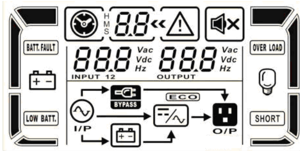
Рисунок 17 – Показания LCD-дисплея ИБП при включении
