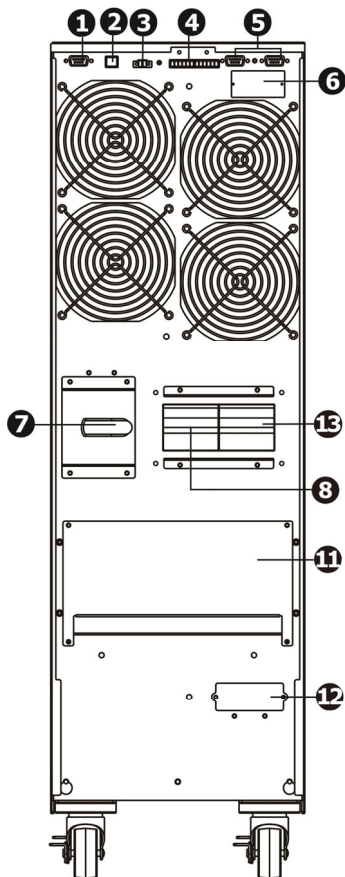
Рисунок 6 - Задняя панель ИБП ATS 30000 3/1 T-X
