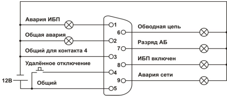
Рисунок 15 – Электрическая схема организации контроля и управления ИБП с электропитанием от источника постоянного тока напряжением +12 В
