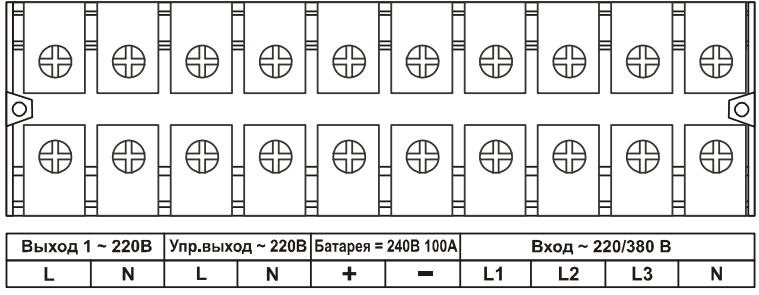
Рисунок 9 – Внешний вид клеммных блоков ИБП ATS 15000 3/1 T-X, ATS 20000 3/1 T-X
