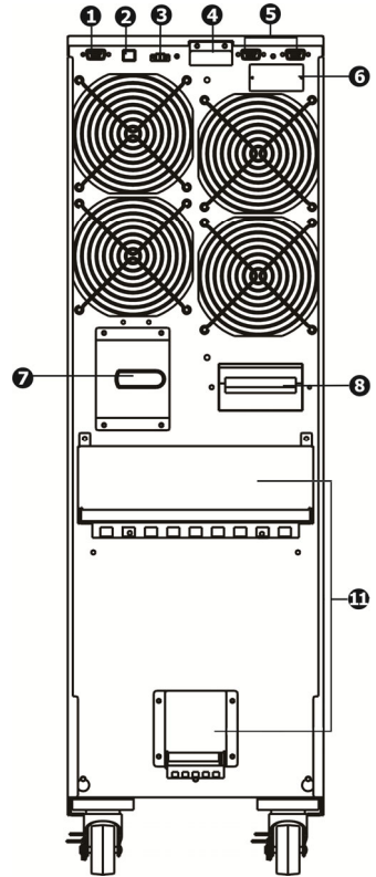
Рисунок 5 - Задняя панель ИБП ATS 15000 3/1 T-BX, ATS 20000 3/1 T-BX
