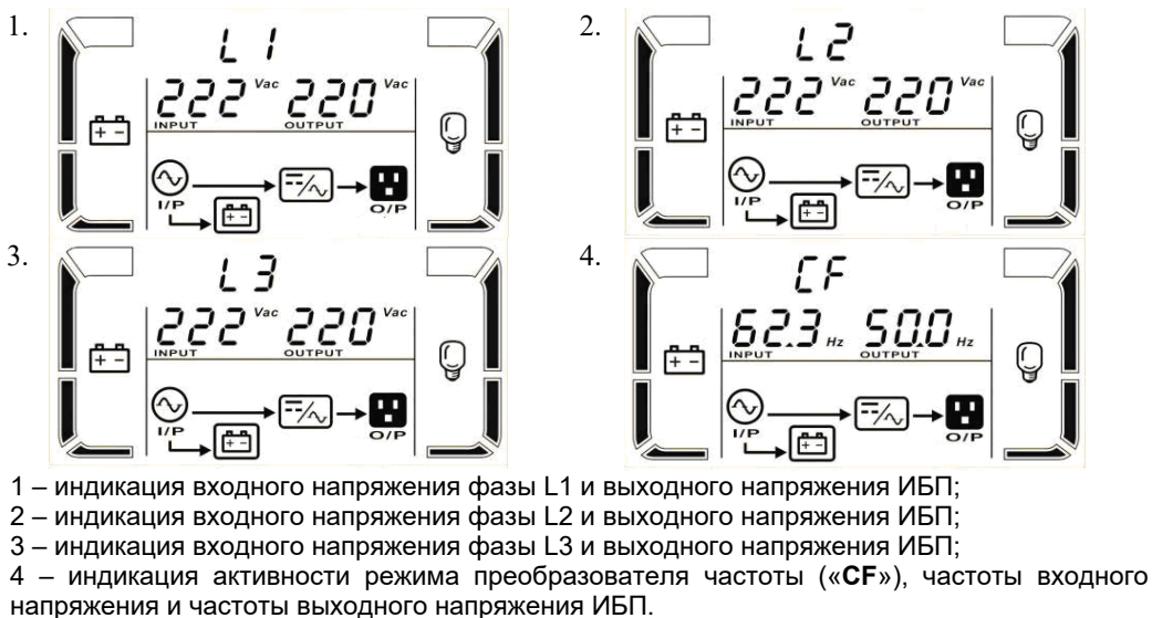
Рисунок 22 – Показания LCD-дисплея ИБП в режиме преобразователя частоты
