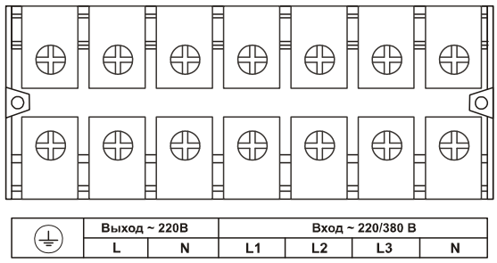
Рисунок 11 – Внешний вид клеммных блоков ИБП ATS 30000 3/1 T-X, ATS 30000 3/1 T-BX
