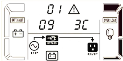
Рисунок 25 – Показания LCD-дисплея ИБП с кодами предупреждающих сообщений
