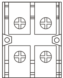
Рисунок 10 – Внешний вид клеммных блоков ИБП ATS 15000 3/1 T-BX, ATS 20000 3/1 T-BX
