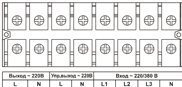
Рисунок 8 – Внешний вид клеммных блоков ИБП ATS 10000 3/1 T-BX, ATS 10000 3/1 T-X
