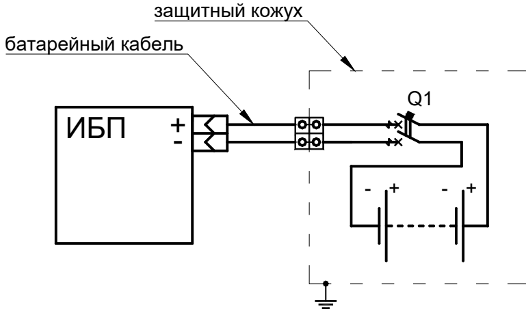
Q1 – автоматический выключатель батареи
