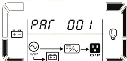
Рисунок 26 – Показания LCD-дисплея при параллельной работе ИБП
