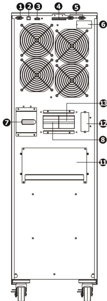
Рисунок 7 - Задняя панель ИБП ATS 30000 3/1 T-BX
