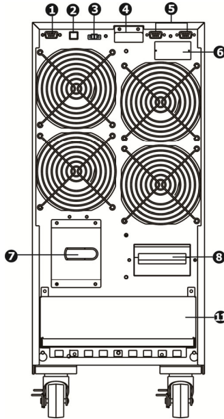
Рисунок 4 - Задняя панель ИБП ATS 15000 3/1 T-X, ATS 20000 3/1 T-X
