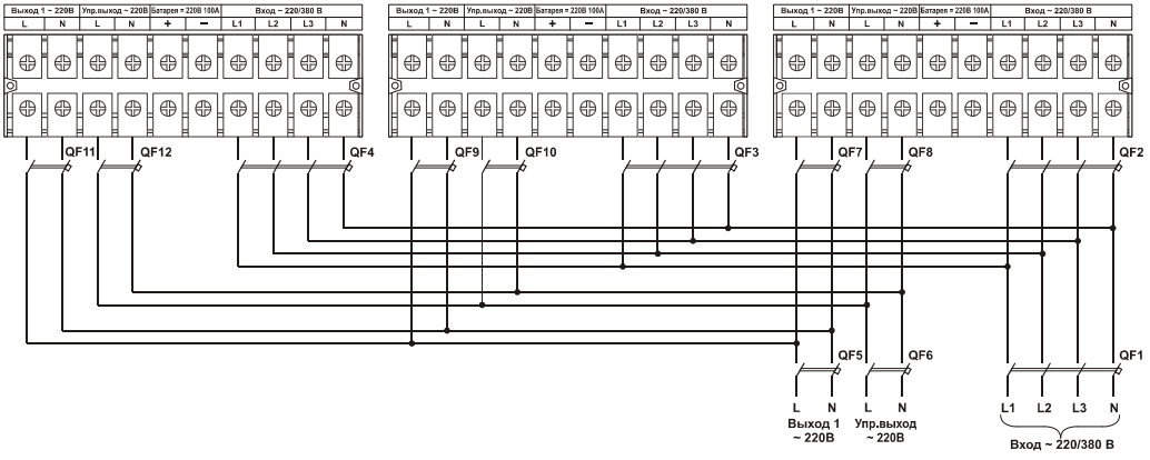
Рисунок 31 – Соединение входов и выходов трех ИБП в параллельной системе
