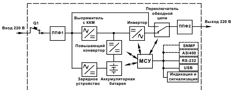
Рисунок 1 - Структурная схема ИБП
