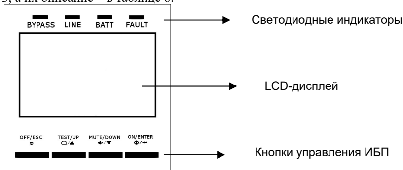
Рисунок 2 – Внешний вид панели управления ИБП
