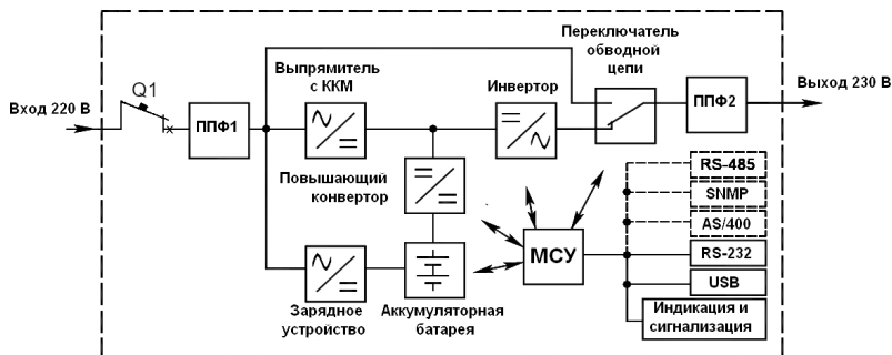
Рисунок 1 - Структурная схема ИБП
