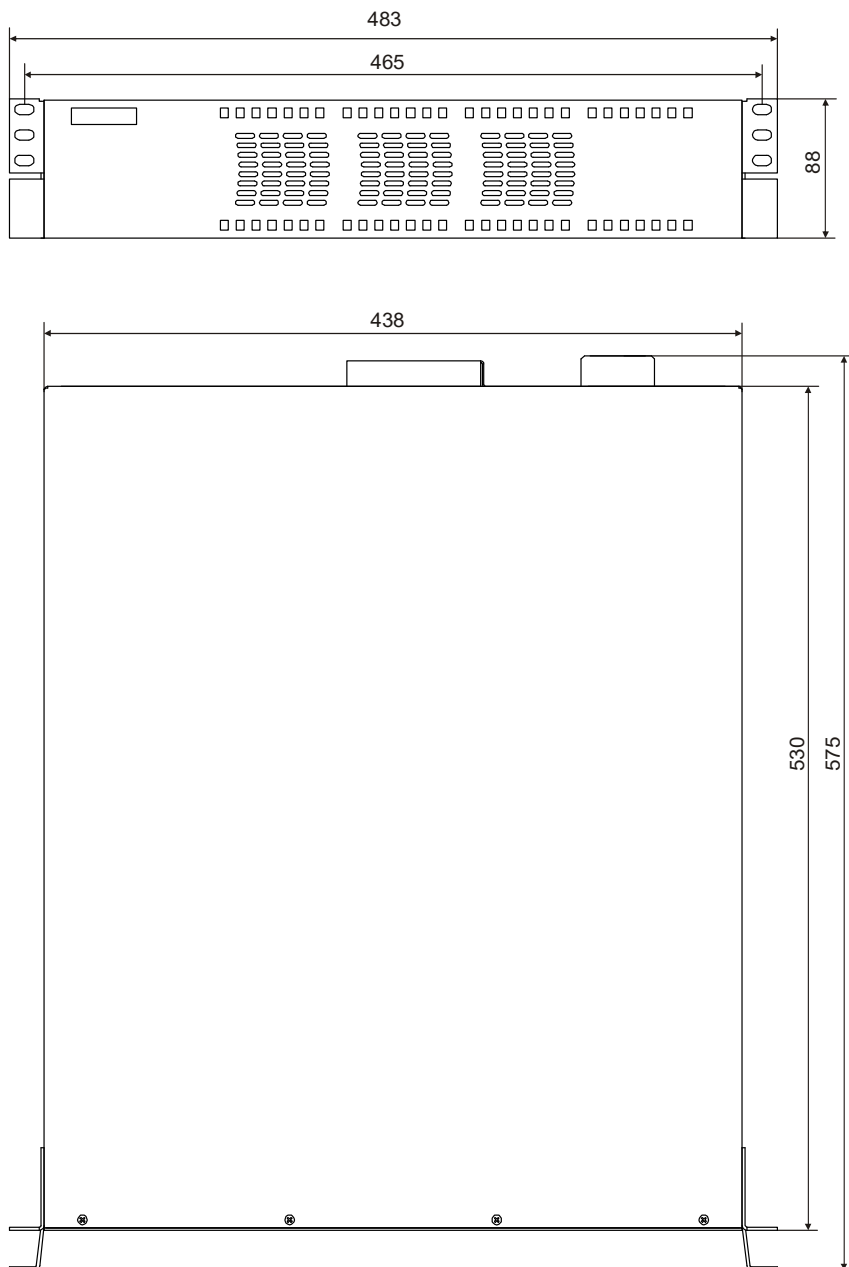
Рисунок А.1 – Габаритные и установочные размеры БМ
