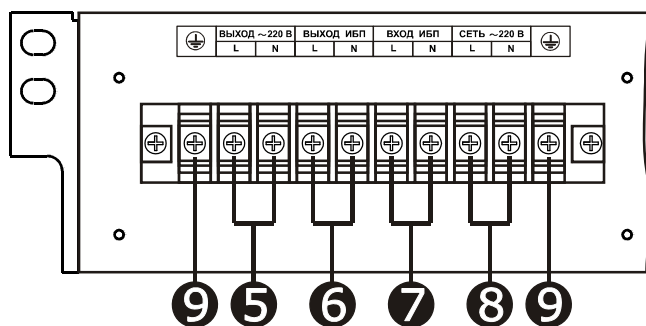
Рисунок 2 – Вид клеммных блоков модуля MBS 1/1 6-10К
