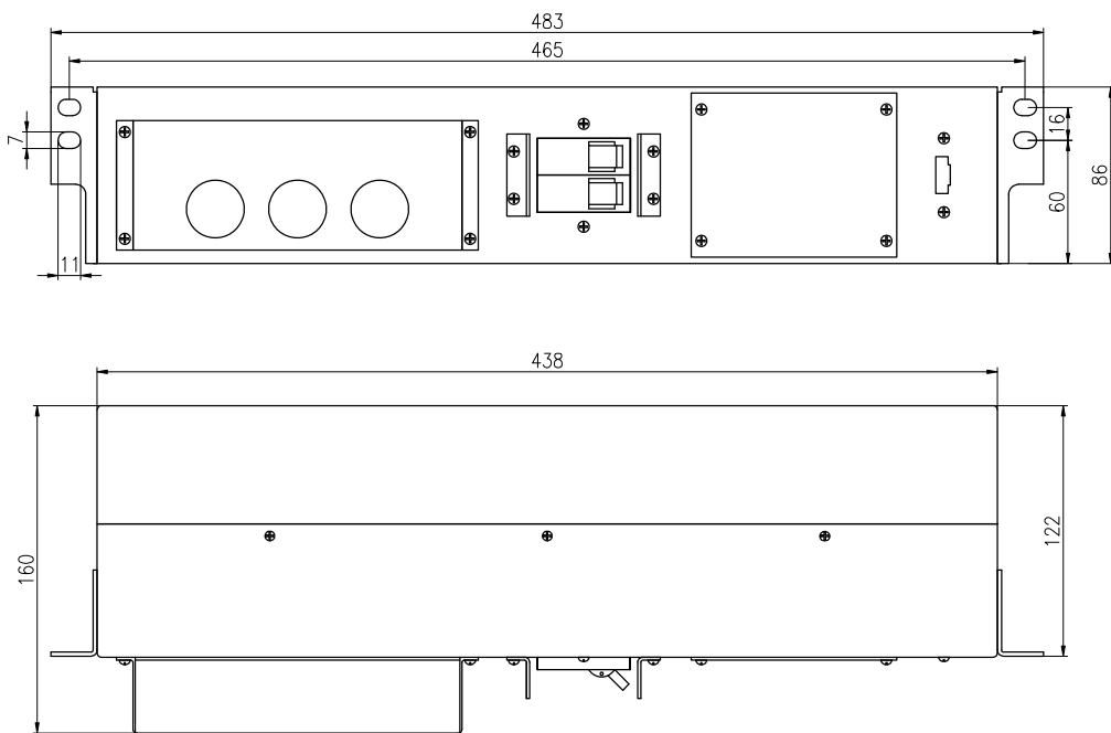
Рисунок А.1 – Габаритные и установочные размеры модуля MBS 1/1 6-10K
