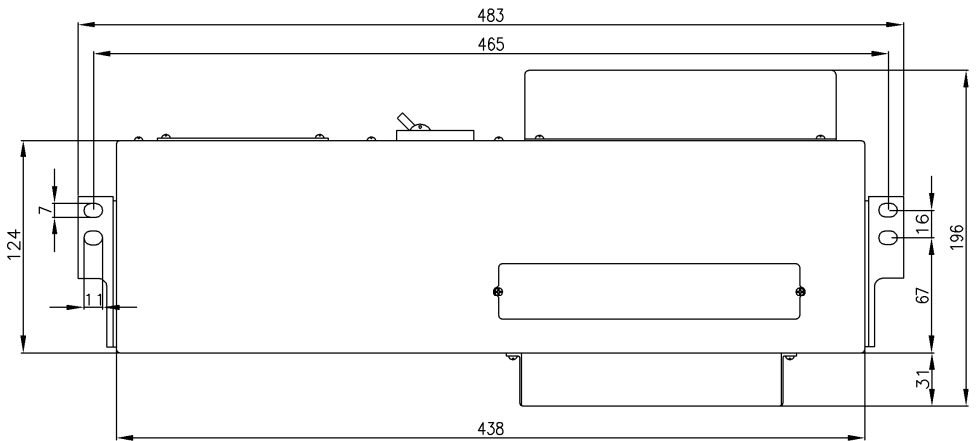
Рисунок А.2 – Установочные размеры модуля MBS 3/1 15-20K при монтаже на стену
