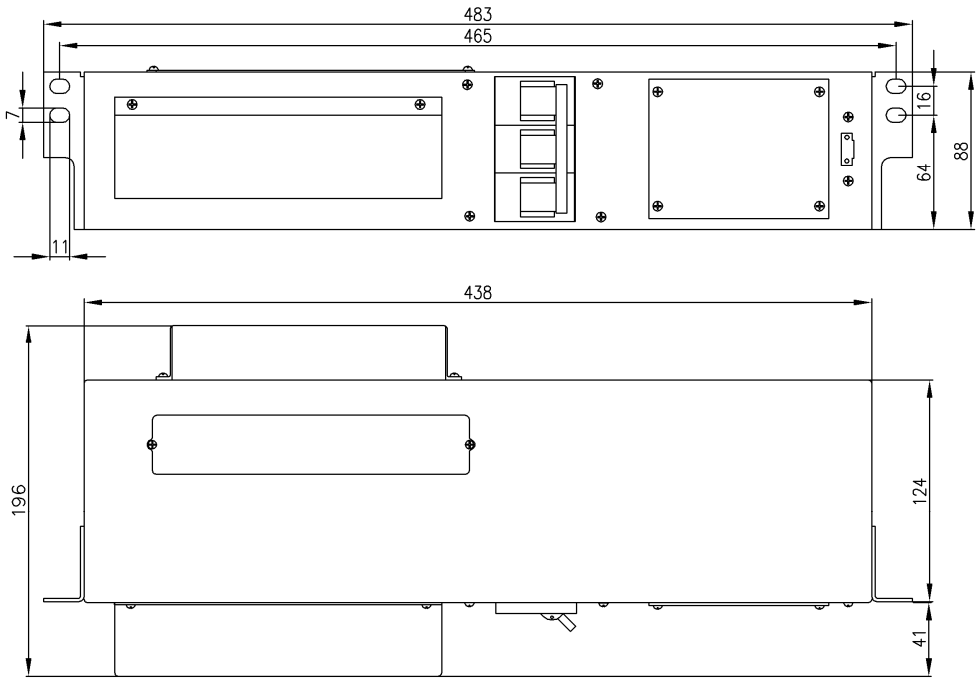
Рисунок А.1 – Габаритные и установочные размеры модуля MBS 3/1 15-20K
