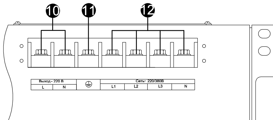
Рисунок 4 – Вид клеммных блоков на задней панели модуля MBS 3/1 15-20К
