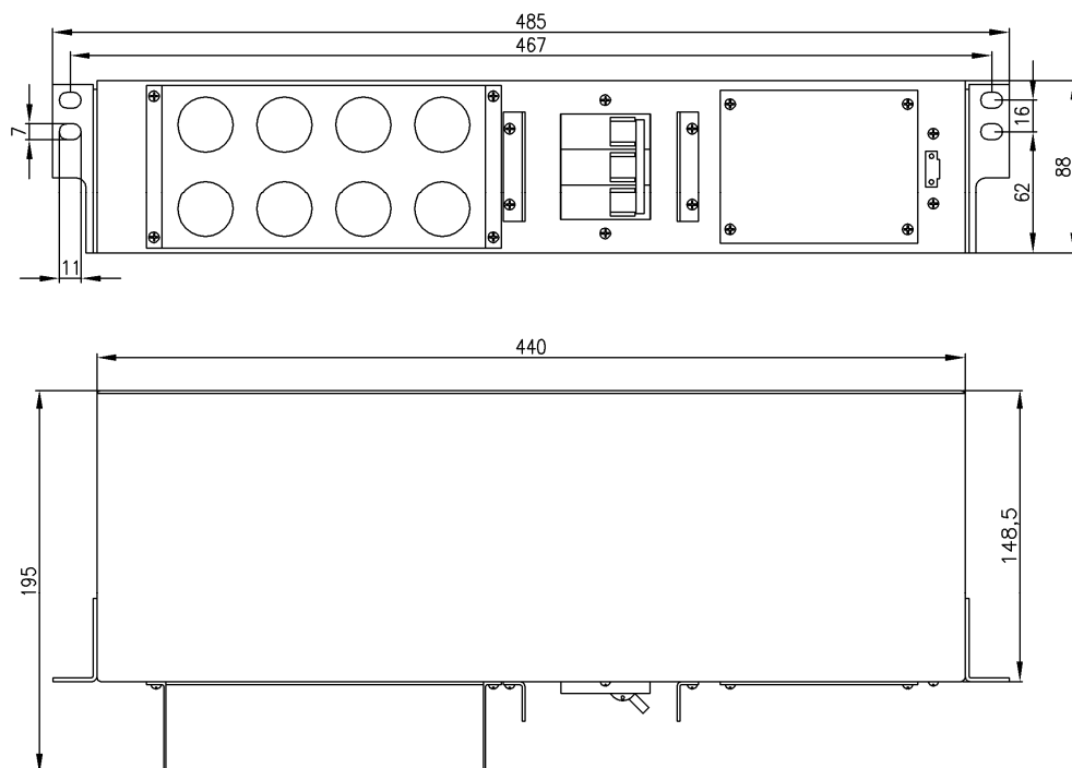
Рисунок А.1 – Габаритные и установочные размеры модуля MBS 3/3 10К
