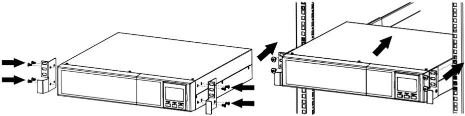
Рисунок 7 – Порядок установки ИБП и БМ в стандартный шкаф или стойку для телекоммуникационного оборудования шириной 19 дюймов
