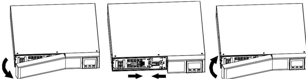
Рисунок 10 – Порядок подключения встроенной батареи ИБП
