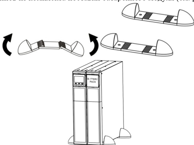
Рисунок 9 – Порядок установки ИБП совместно с БМ в вертикальное напольное (настольное) положение
