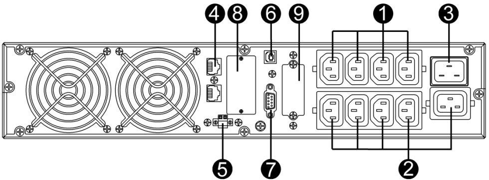
Рисунок 6 - Задняя панель ИБП ATS 3000 R-E, ATS 3000 R-BE
