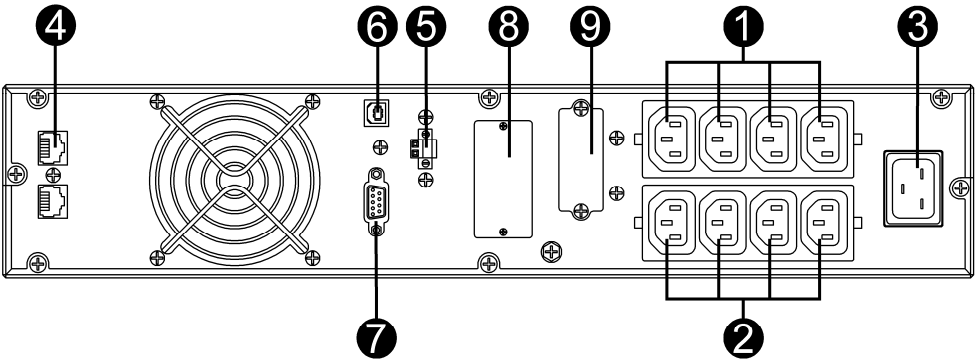
Рисунок 5 – Задняя панель ИБП ATS 2000 R-E, ATS 2000 R-BE
