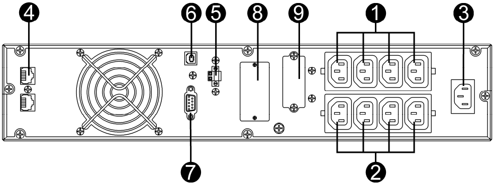
Рисунок 4 – Задняя панель ИБП ATS 1000 R-E, ATS 1000 R-BE, ATS 1500 R-E, ATS 1500 R-BE
