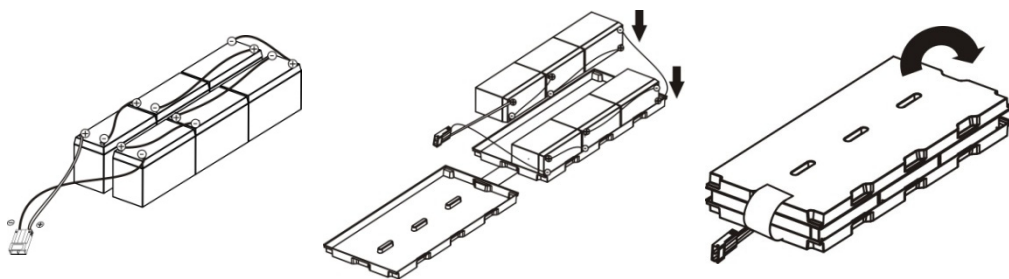
Рисунок 18 – Последовательность установки аккумуляторов в контейнер ИБП ATS 3000 R-VE
