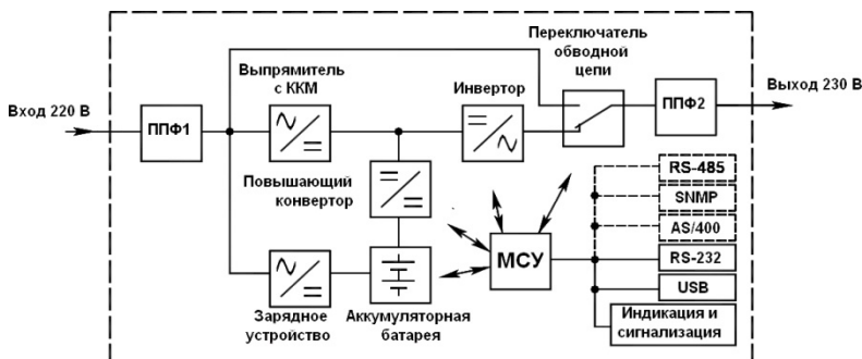
Рисунок 1 - Структурная схема ИБП
