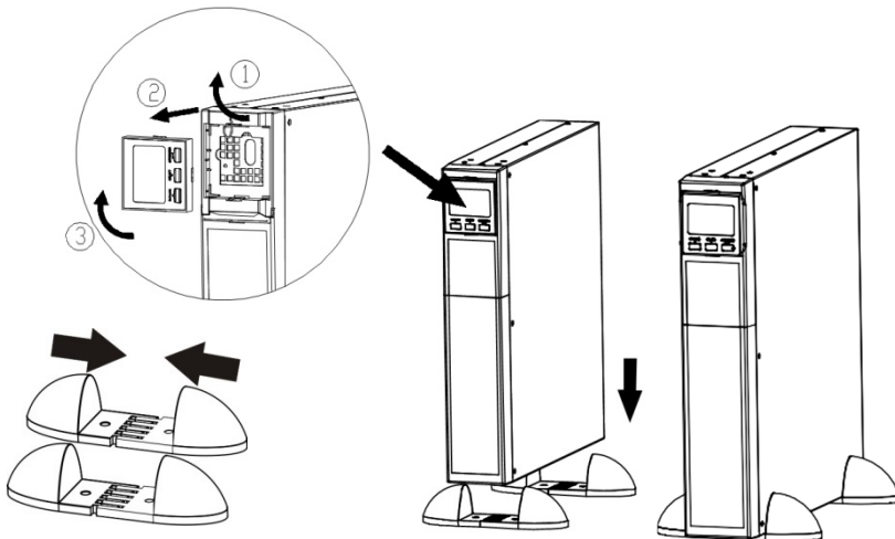
Рисунок 8 – Порядок установки ИБП в вертикальное напольное (настольное) положение
