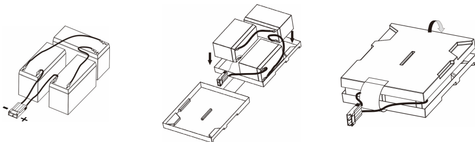
Рисунок 16 – Последовательность установки аккумуляторов в контейнер ИБП ATS 1000 R-VE, ATS 1500 R-VE
