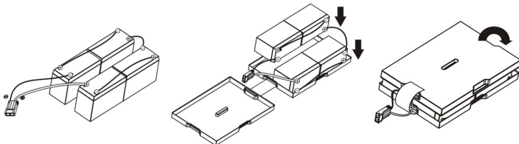
Рисунок 17 – Последовательность установки аккумуляторов в контейнер ИБП ATS 2000 R-VE
