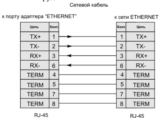
Рисунок 2 - Схема электрическая сетевого кабеля Ethernet 100Base-TX/10Base-T
