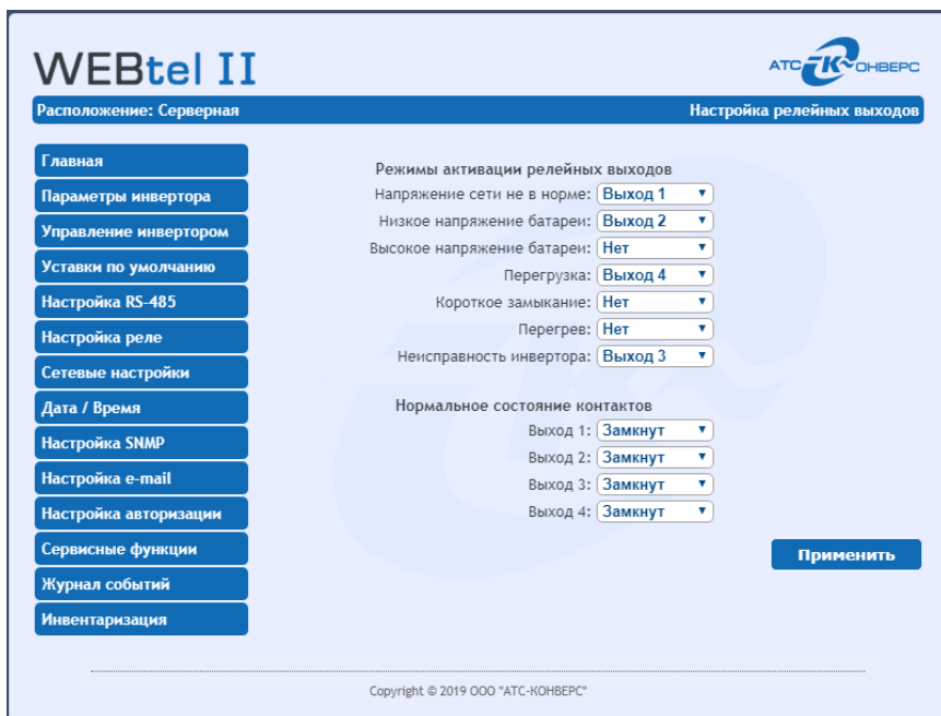
Рисунок 12 – Страница настройки релейных выходов
