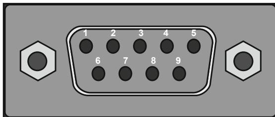
Рисунок 22 – Нумерация контактов разъема порта RS-232 адаптера
